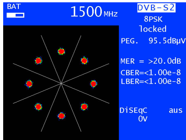
Ideales Konstellationsdiagramm > Signalquelle SFU (Rohde & Schwarz)
