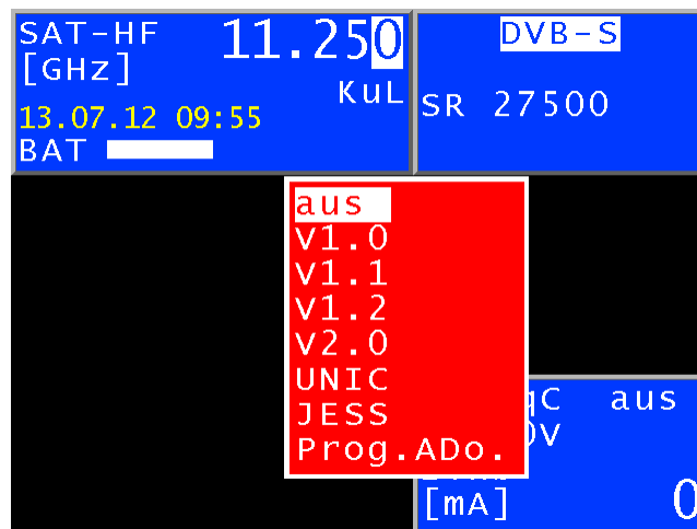
Die Abbildung zeigt das Auswahlmenü für die DiSEqC-Versionen und Einkabel-Standards.
