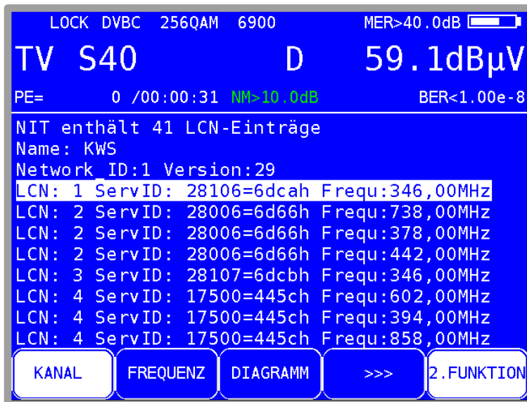
Abbildung 13-4 LCN-Liste
