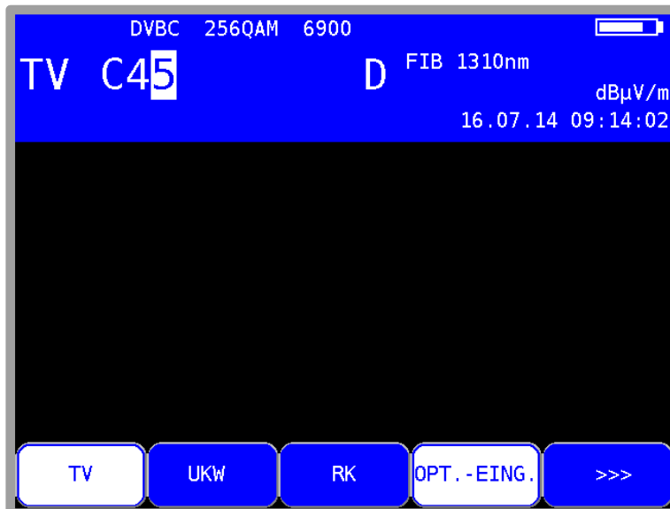
Abbildung 18-1 Optischer Eingang
