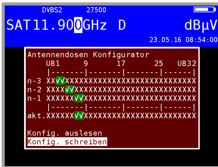
Abbildung 7-23 Antennendosen Konfigurator
