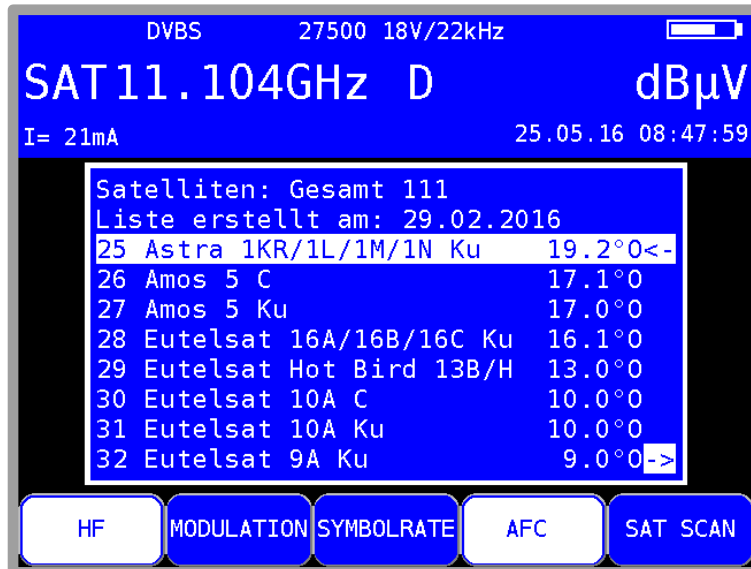
Abbildung 17-3 SAT-Liste
