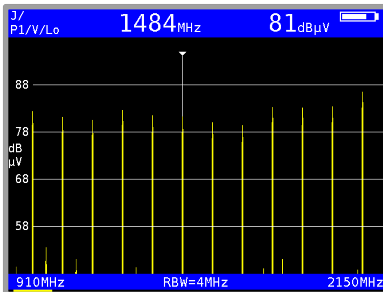
Abbildung 7-28 Testbaken
