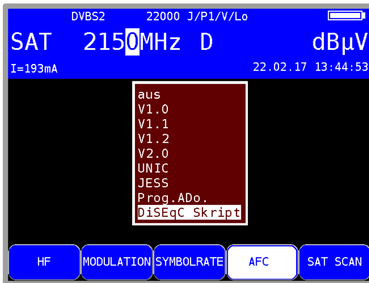
Abbildung 7-13 DiSEqC Menü
