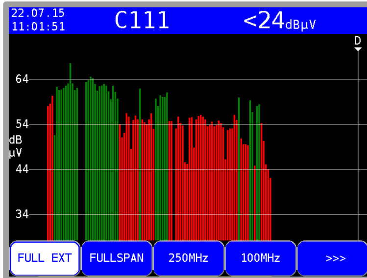
Abbildung 16-2 Spektrumanalyzer Bandbreitenauswahl
