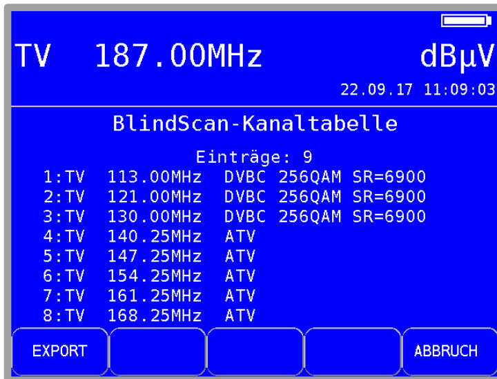
Abbildung 8-22 BlindScan-Kanaltabelle
