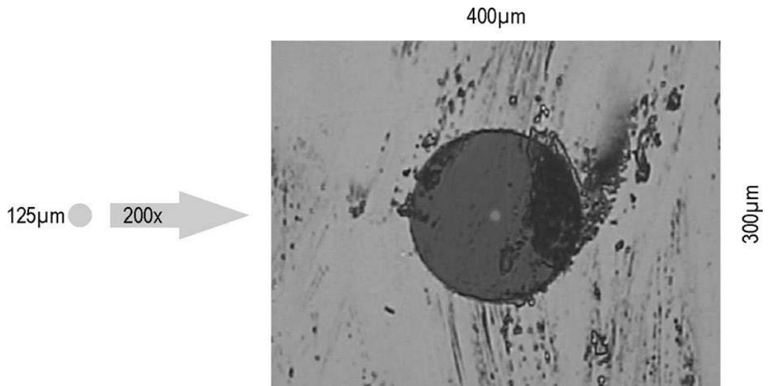
Abbildung 18-6 Mikroskop Vergrößerung
