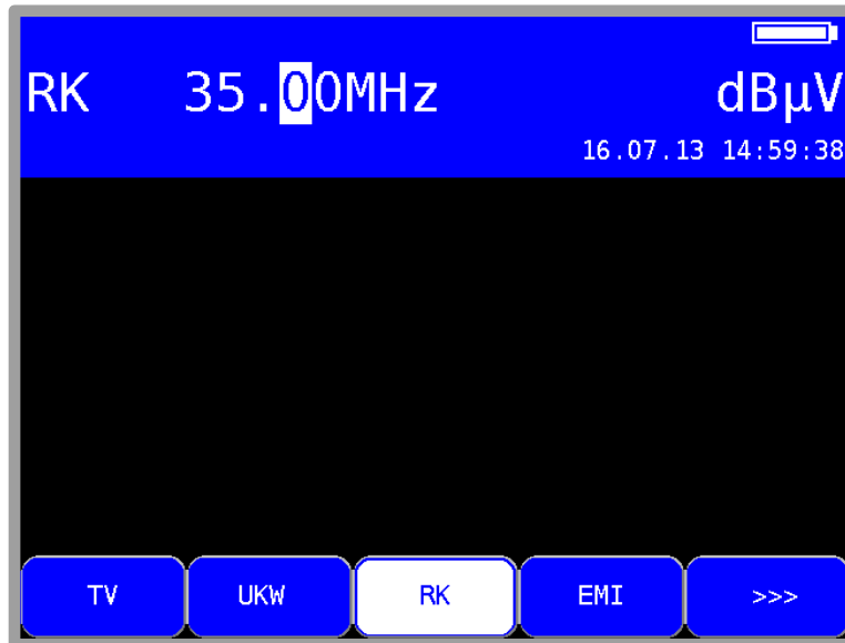
Abbildung 10-1 RK Messbereich
