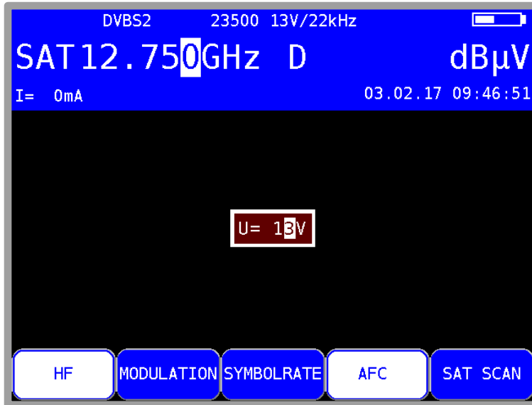
Abbildung 7-10 LNB-Spannung einstellen
