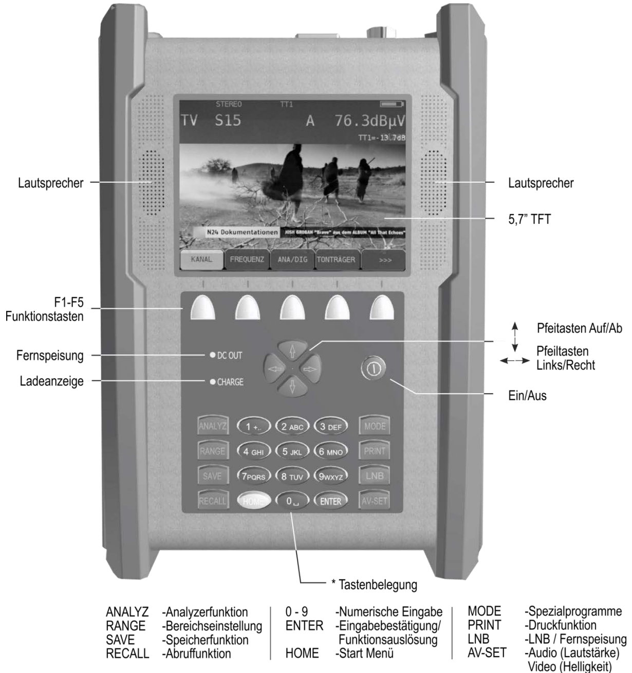
Abbildung 4-1 Gerätefrontseite
