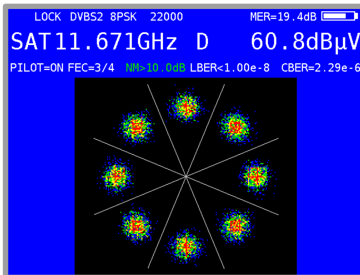
Abbildung 14-6 DVBS-2 Konstellationsdiagramm
