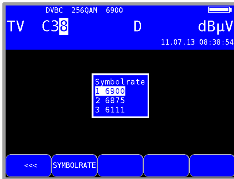
Abbildung 8-5 Symbolraten-Einstellung
