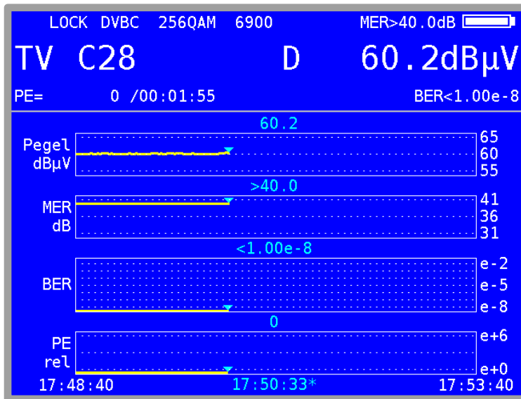
Abbildung 21-2 DataGrabber Aufzeichnung
