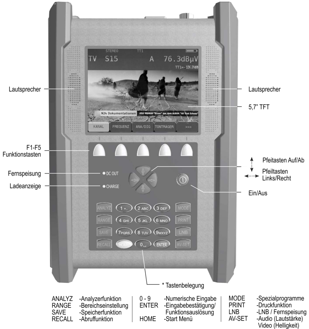
Abbildung 4-1 Gerätefrontseite
