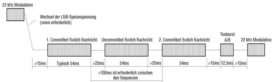
Abbildung 7-13 DiSEqC V1.1 Steuerablauf mit Wiederholung
