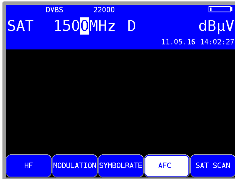
Abbildung 7-1 SAT Grundzustand ZF
