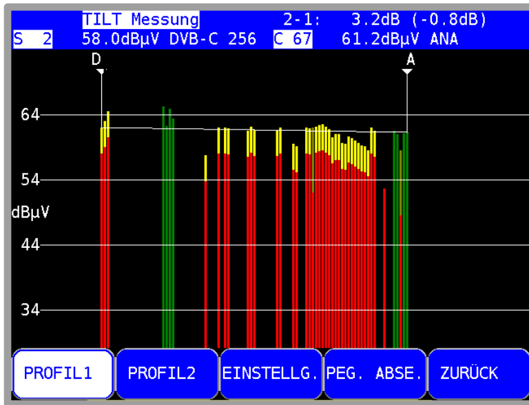
Abbildung 16-4 Schräglagenmessung TILT
