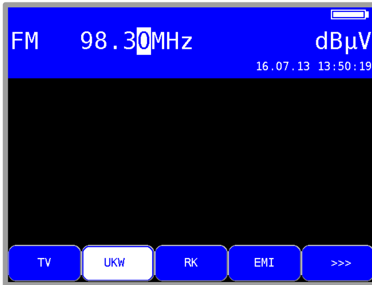
Abbildung 9-1 UKW Messbereich
