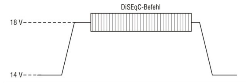
Abbildung 7-16 UNICABLE Befehl
