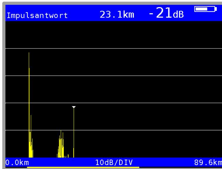
Abbildung 8-14 DVB-T Impulsantwort
