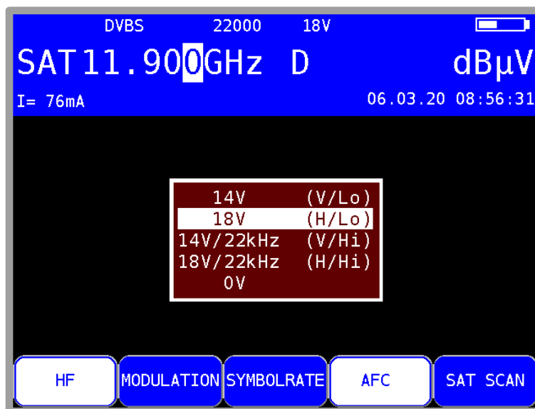
Abbildung 7-7 SAT-ZF-Ebene
