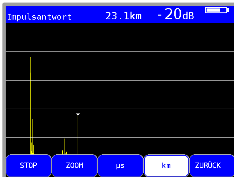
Abbildung 8-13 DVB-T Impulsantwortmenü
