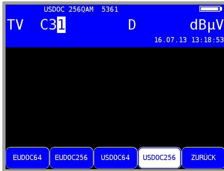
Abbildung 8-8 DOCSIS-Modulationsart
