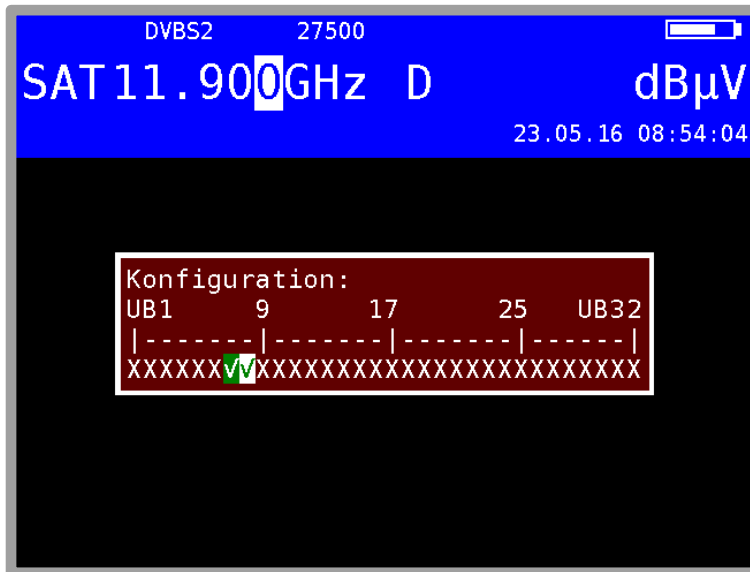
Abbildung 7-22 UBs konfigurieren
