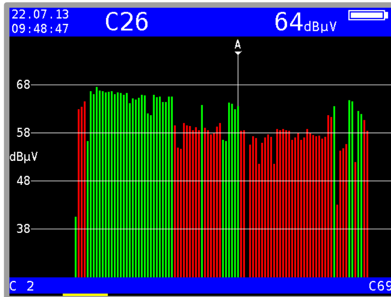
Abbildung 16-3 Pegeldiagramm
