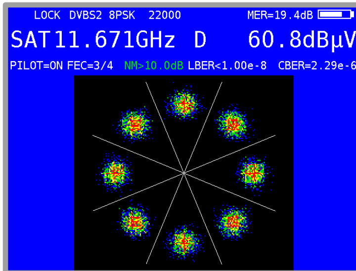
Abbildung 14-6 DVBS-2 Konstellationsdiagramm
