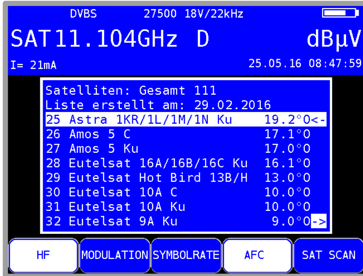
Abbildung 17-3 SAT-Liste
