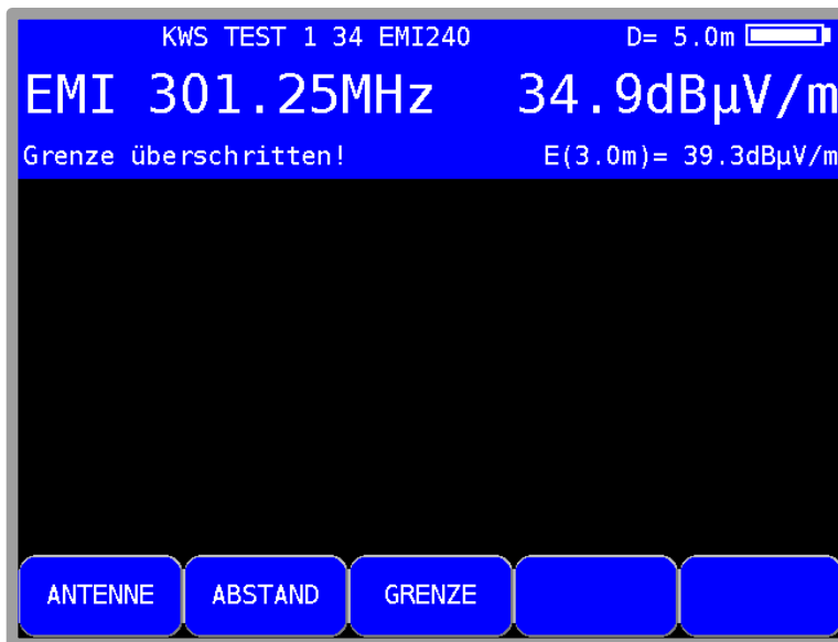
Abbildung 12-3 Störstrahl Feldstärkenmessung
