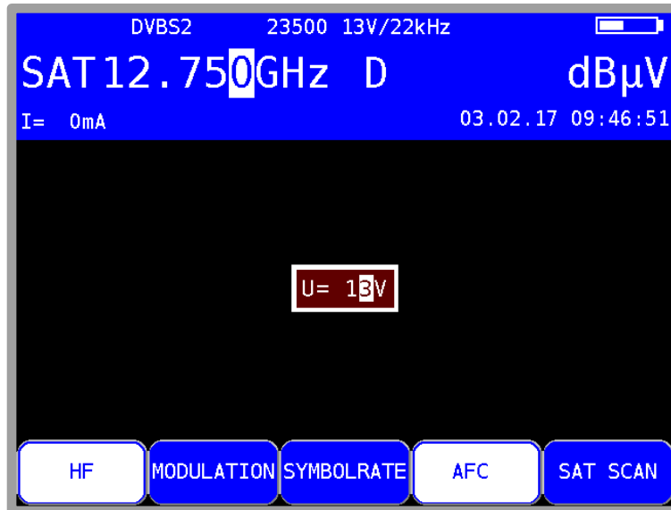
Abbildung 7-8 LNB-Spannung einstellen
