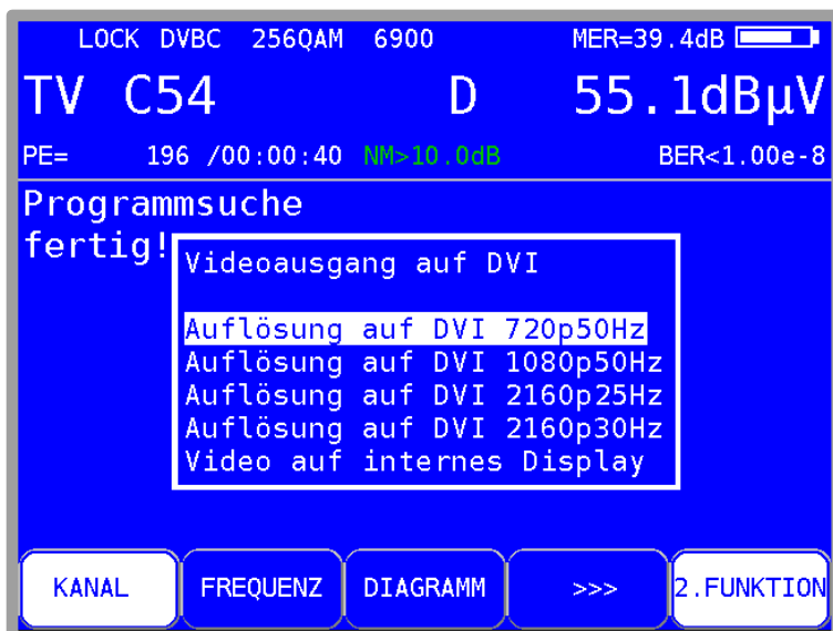
Abbildung 22-2 Videoauflösung bei HDTV über DVI über DVI Auswahlmenü
