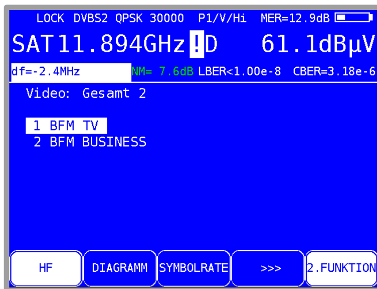
Abbildung 7-6 SAT Frequenzoffset anzeigen
