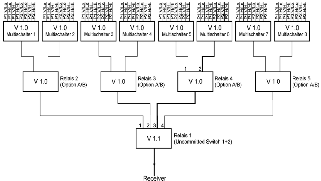
Abbildung 7-14 DiSEqC V1.1 Aufbau mit 64 SAT-ZF Ebenen
