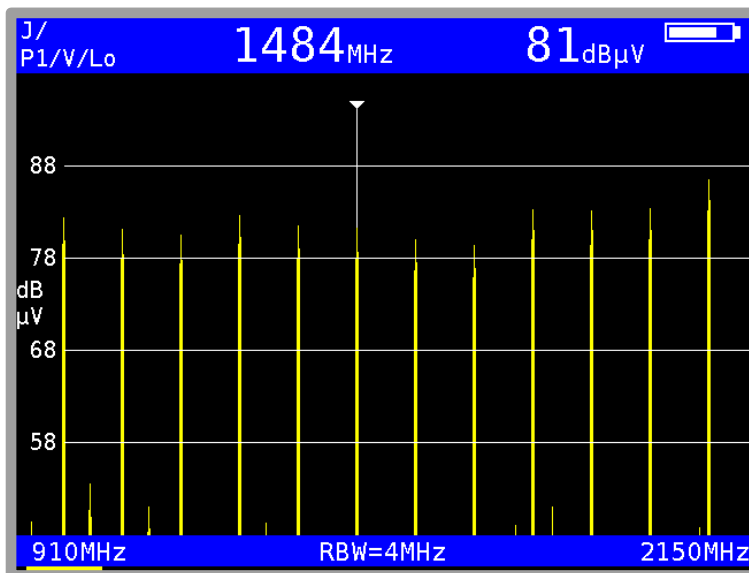
Abbildung 7-26 Testbaken
