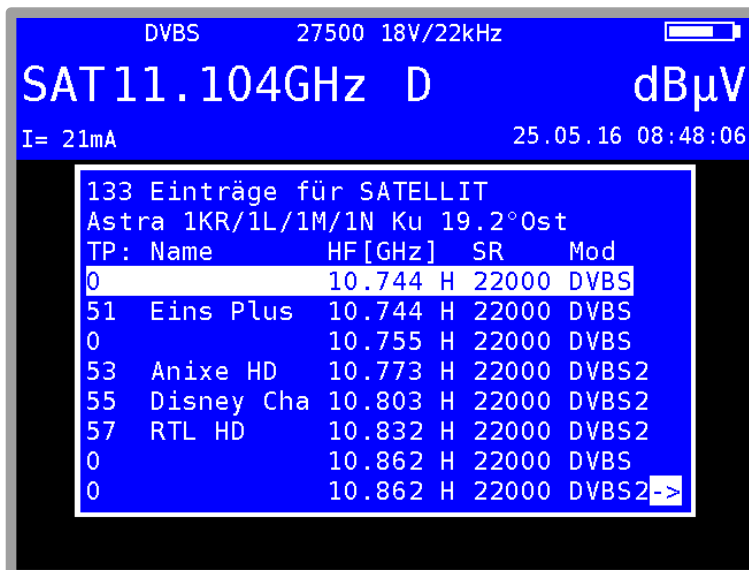
Abbildung 17-4 Transponder-Liste
