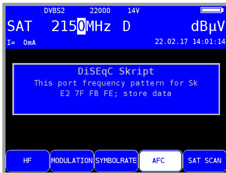
Abbildung 7-27 DiSEqC Skript
