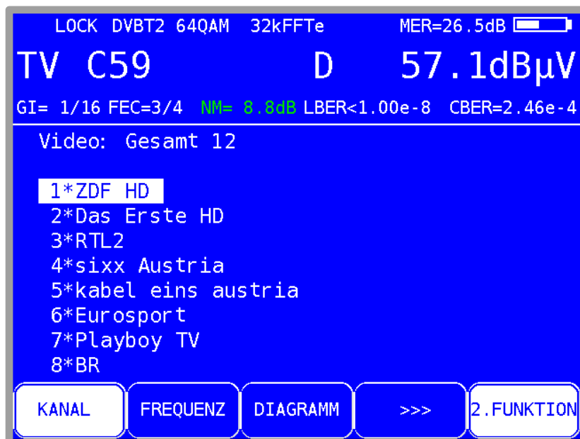
Abbildung 8-17 DVB-T2 Messung
