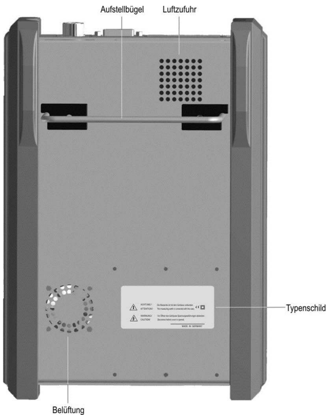
Abbildung 4-2 Geräterückseite
