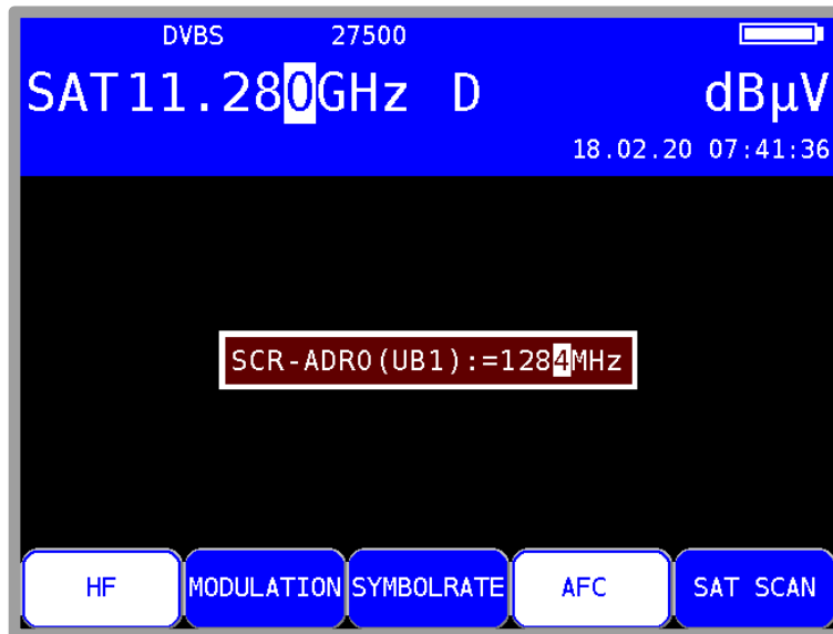
Abbildung 7-18 UNICABLE SCR-ADR editieren
