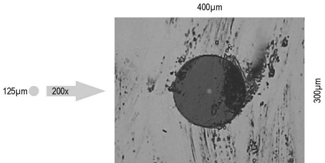
Abbildung 18-6 Mikroskop Vergrößerung
