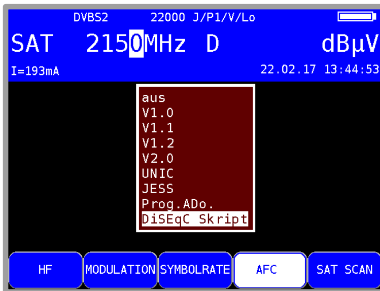
Abbildung 7-11 DiSEqC Menü
