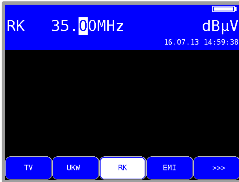
Abbildung 10-1 RK Messbereich
