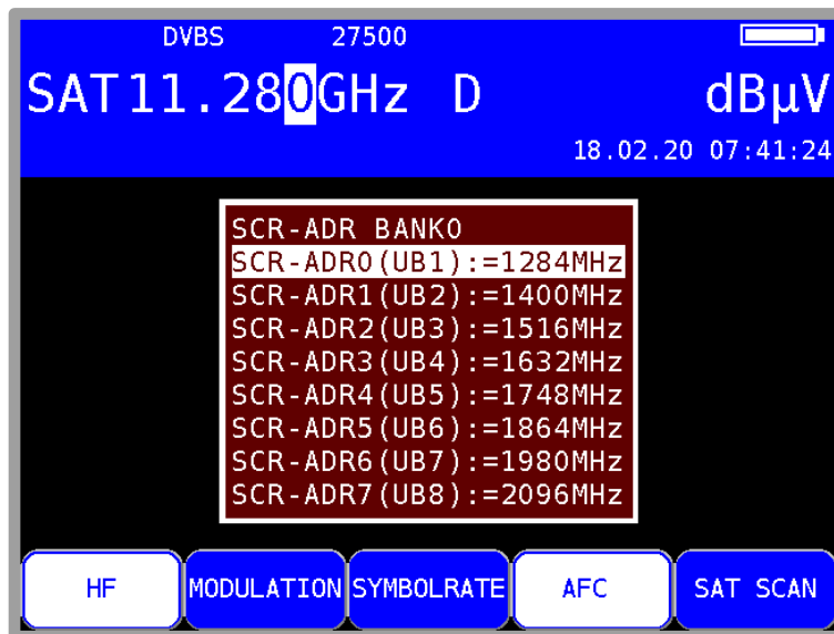
Abbildung 7-17 UNICABLE SCR-ADR aktivieren
