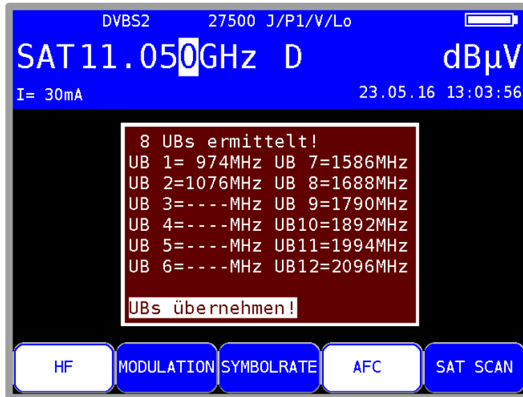
Abbildung 7-24 UB-Scheibenfrequenzen von CSS lesen
