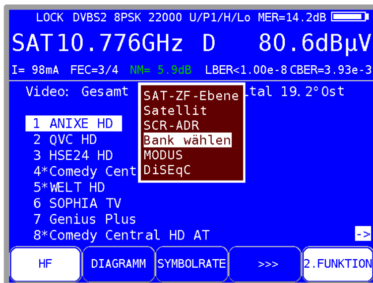
Abbildung 7-20 UNICABLE LNB-Menü
