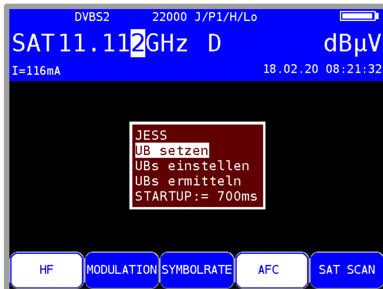
Abbildung 7-23 JESS aktivieren und UBs einstellen
